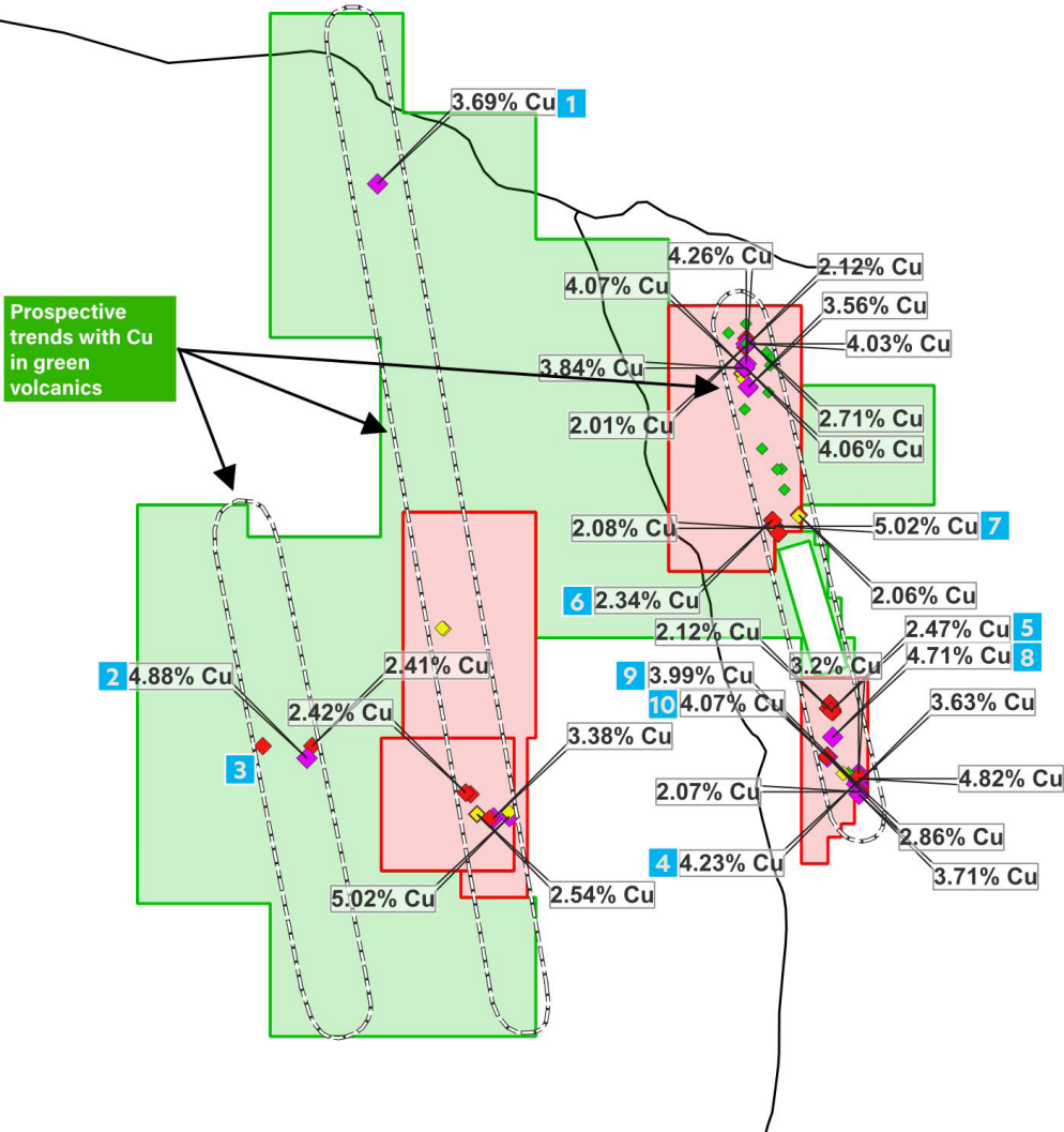
ROS 119 - 2.34% Cu
